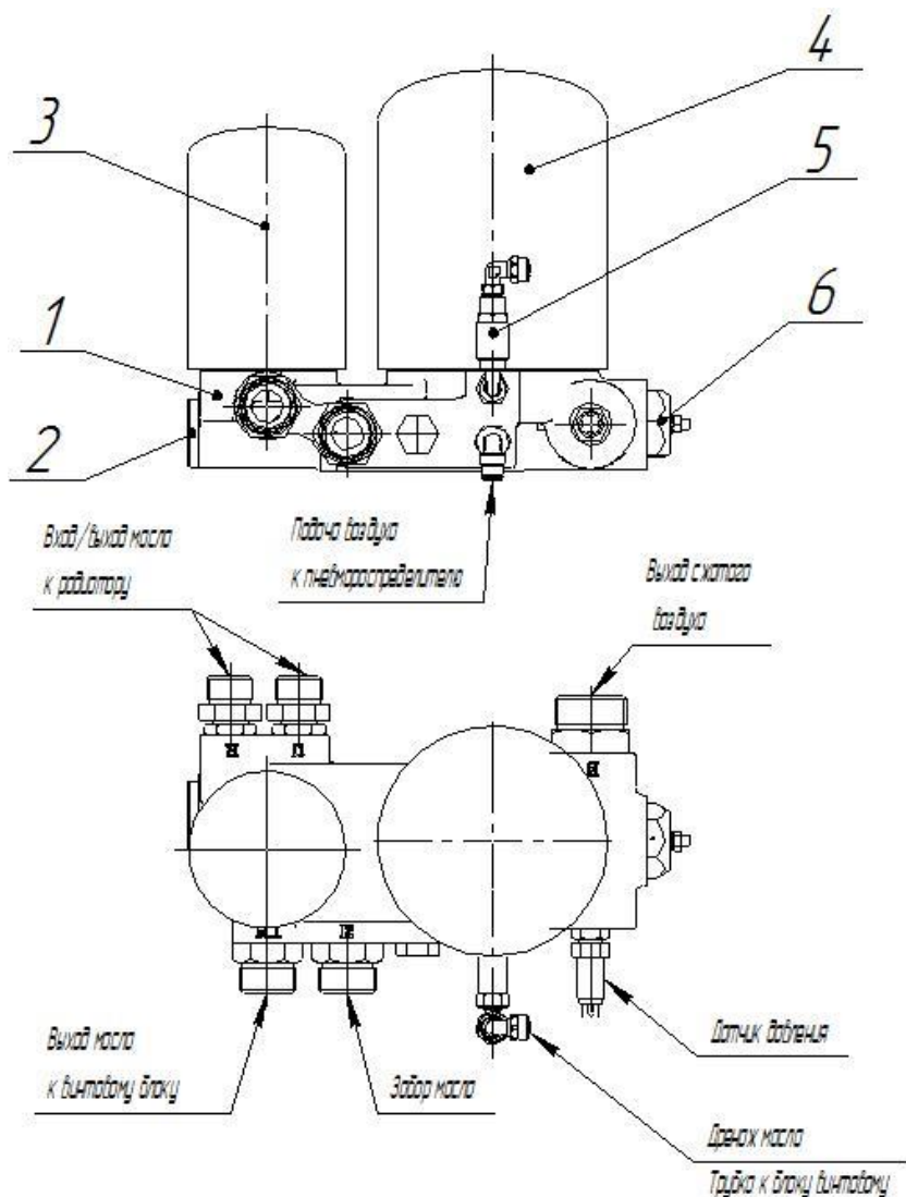
Рисунок 7. Мультиблок
