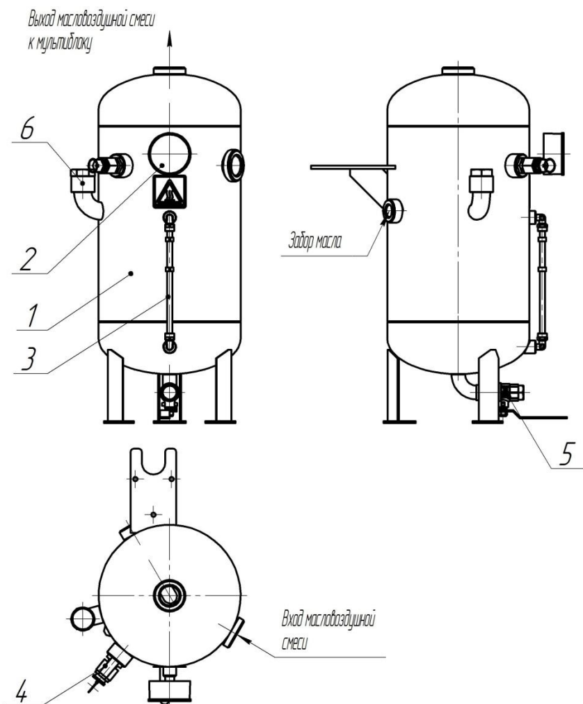
Рисунок 5. Маслоотделитель
