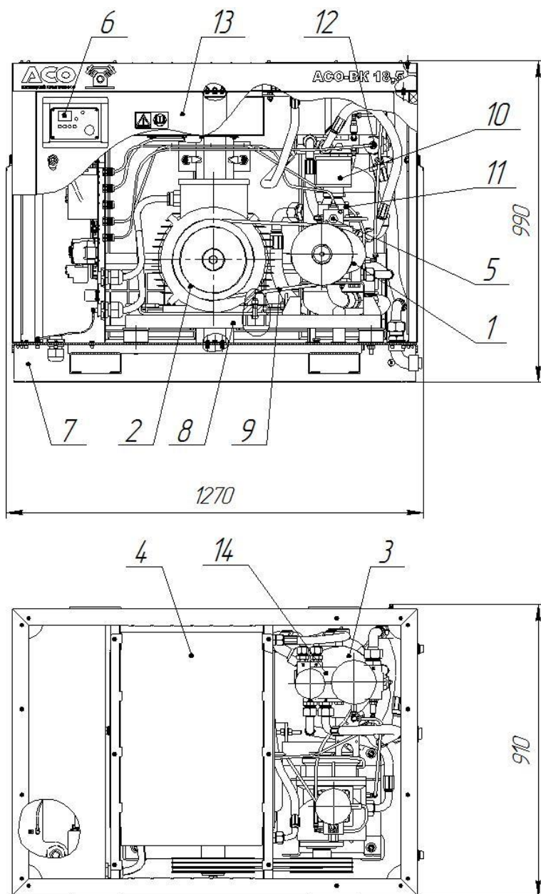
Рисунок 2. Агрегат компрессорный.
